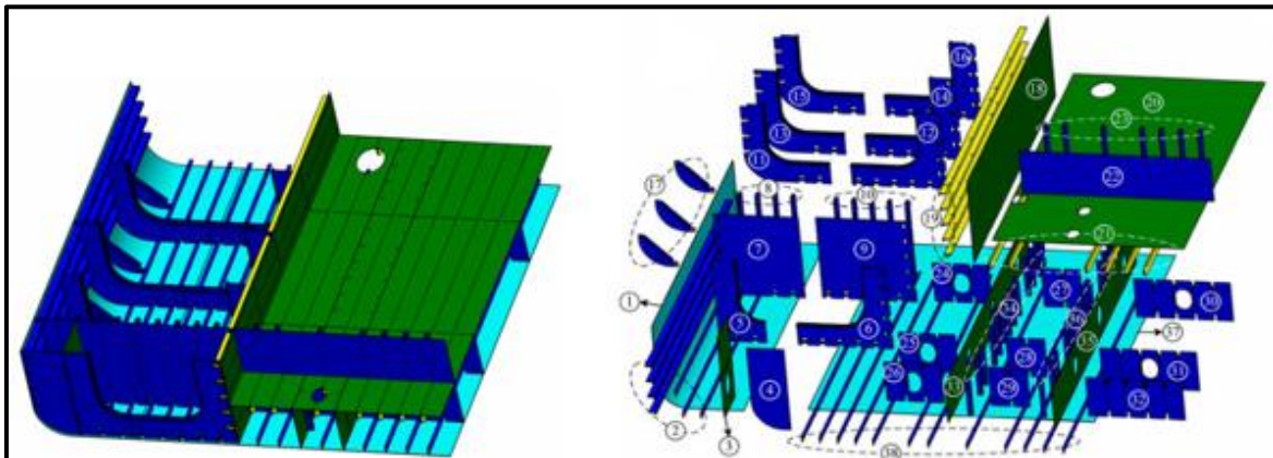
Figure 2: Hull block (Bertram et al. 2005)
